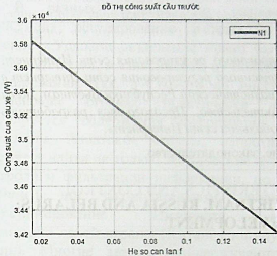
Hình 4. Đồ thị công suất của cầu trước phụ thuộc vào hệ số cản lăn.
