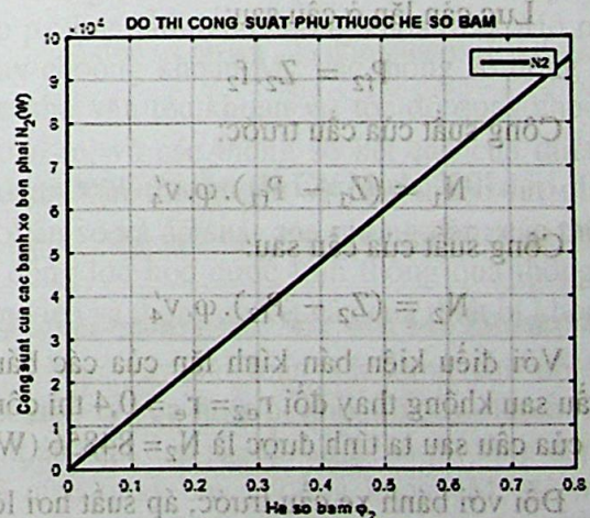
Hình 2. Đồ thị công suất của các bánh xe bên phải.
