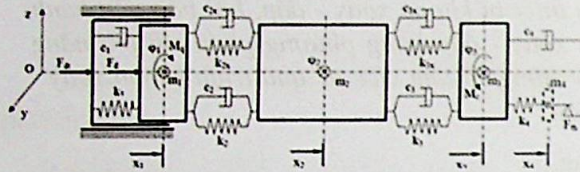
Hình 1. Mô hình động lực học khoan xoay đập.
