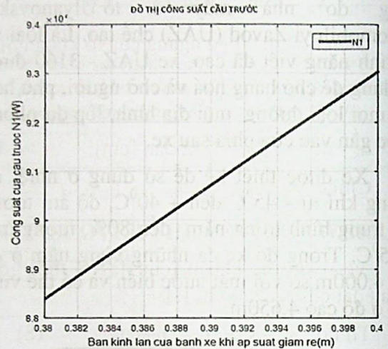
Hình 3. Đồ thị công suất của cầu trước phụ thuộc vào bán kính lăn.
