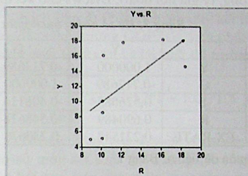
Đồ thị 2. (Y) vs. Lãi suất thị trường (R)
